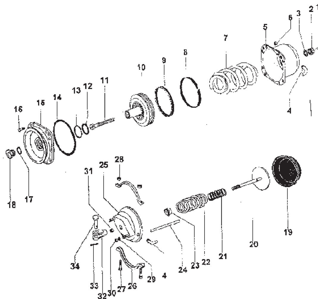
REAR BRAKE ACTUATOR (S-CAM)
