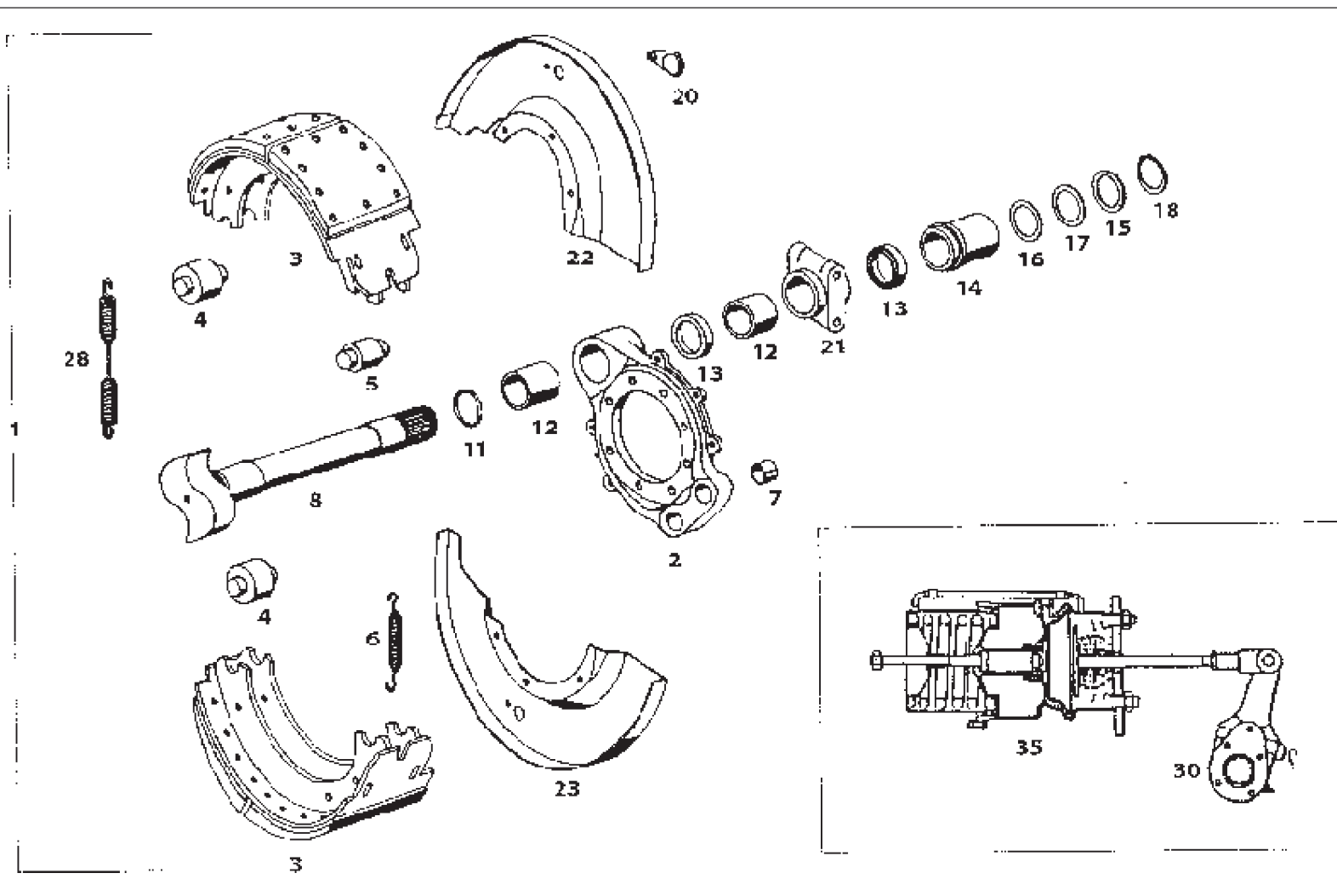
BRAKE ASSY. REAR (S-CAM) (BIL)
