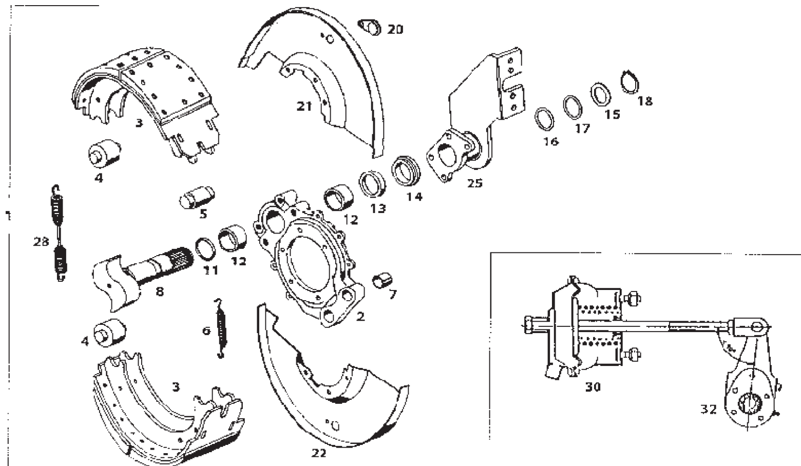
BRAKE ASSY. FRONTS (S-CAM) (BIL)
